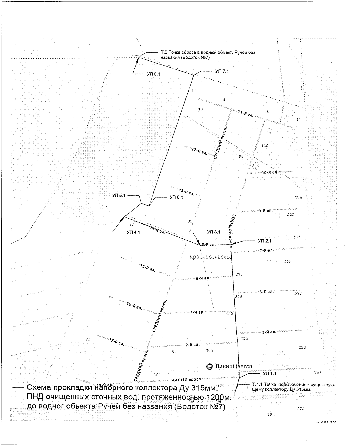
Рисунок 1. Ситуационный план подключения объекта заявителя к централизованной системе водоотведения ООО «PCO-ЮГ»
